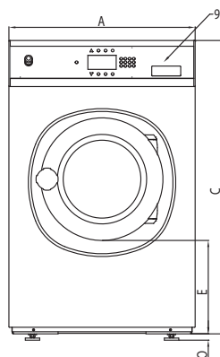
Frente
