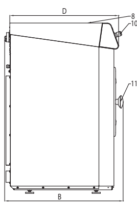
Lado esquerdo
